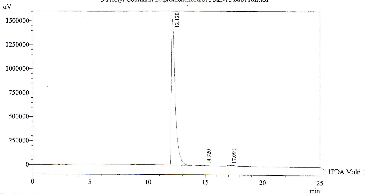
Chromatogram 3-Acetyl Coumarin D:\promonence\2010\Jan-10\080110B.lcd
